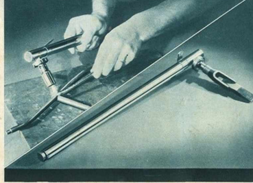
Vue du "PIP" muni du fer et lampe à souder (Dimensions : 47 x 16 mm)
